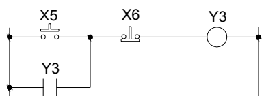
傳統階梯圖
